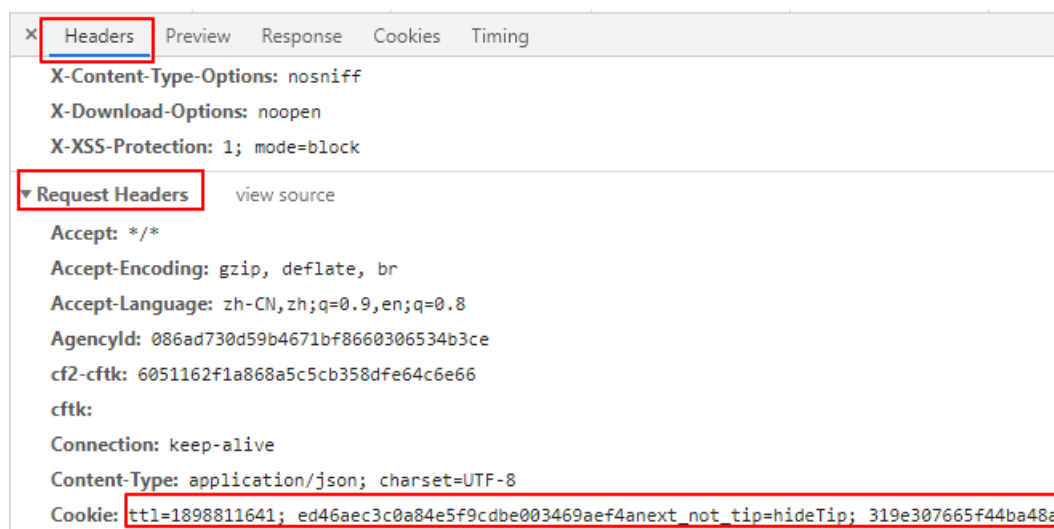
图 2-7 获取 cookie 值
