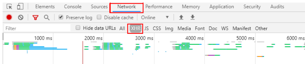
图 2-6 Network 页面
